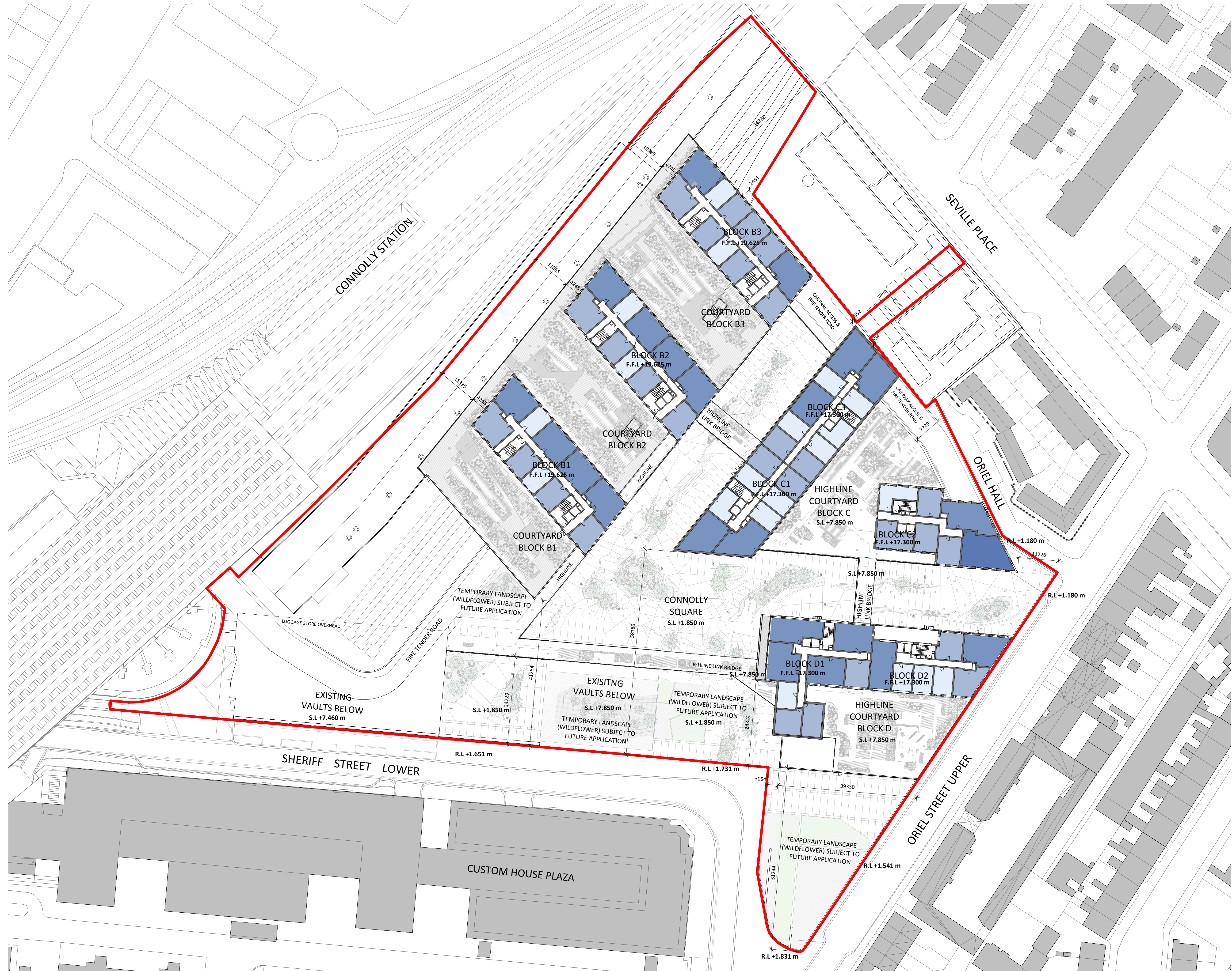
1 SITE LAYOUT PLAN - LEVEL 04 1 : 500
